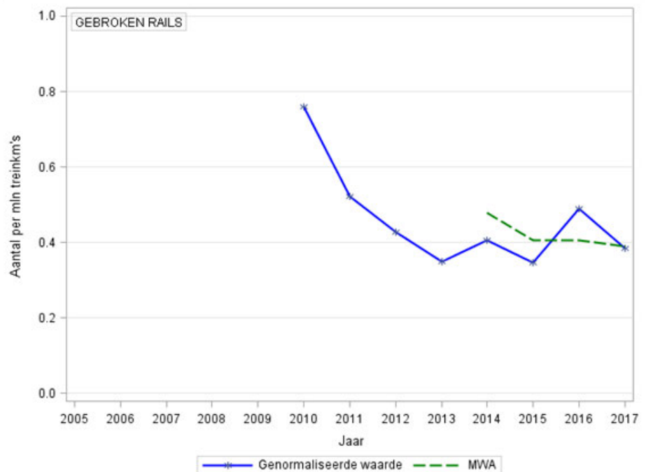
Figuur 15: Trend in het genormaliseerde aantal (op basis van miljoen treinkilometers) en de MWA van het aantal gebroken rails over de jaren 2005-2017.
