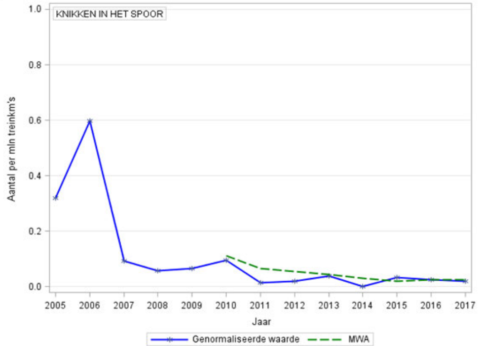
Figuur 16: Trend in het genormaliseerde aantal (op basis van miljoen treinkilometers) en de MWA van het aantal spoorspattingen (knikken in het spoor) over de jaren 2005-2017.
