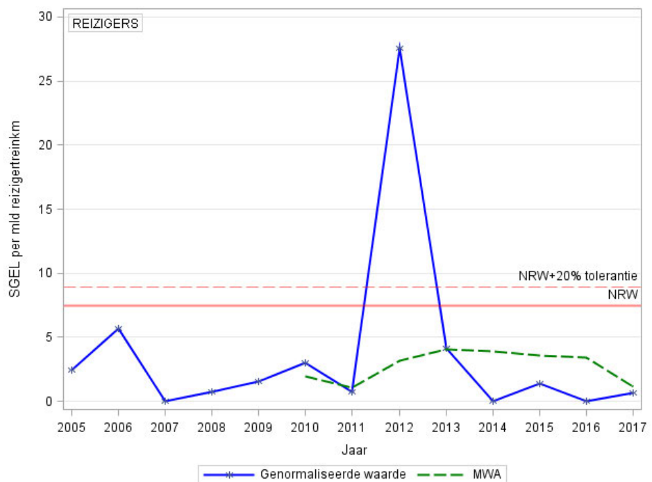
Figuur 5: Trend in de genormaliseerde SGEL (op basis van miljard reizigerreïnkilometers) en de MWA van reizigers over de jaren 2005-2017.
