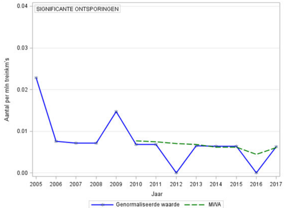
Figuur 14: Trend in het genormaliseerde aantal (op basis van miljoen treinkilometers) en de MWA van het aantal significante ontsporingen over de jaren 2005-2017.
