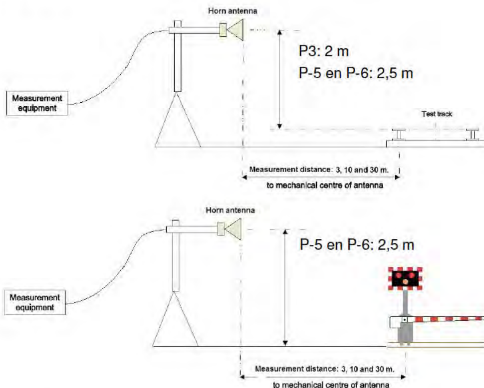
Figuur 4.4-1: Testopstellingen.
