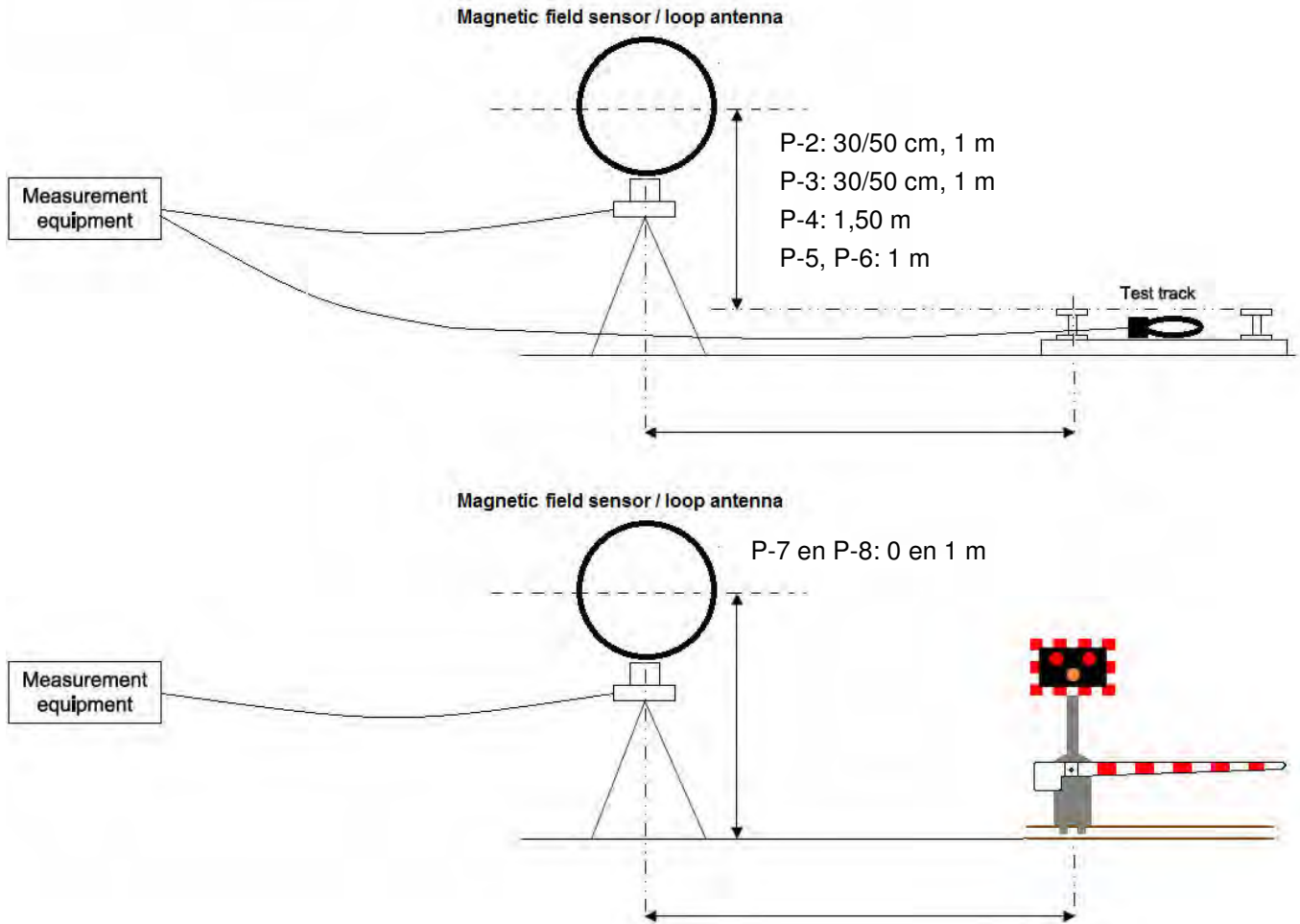
Figuur 4.2-1: Testopstellingen
