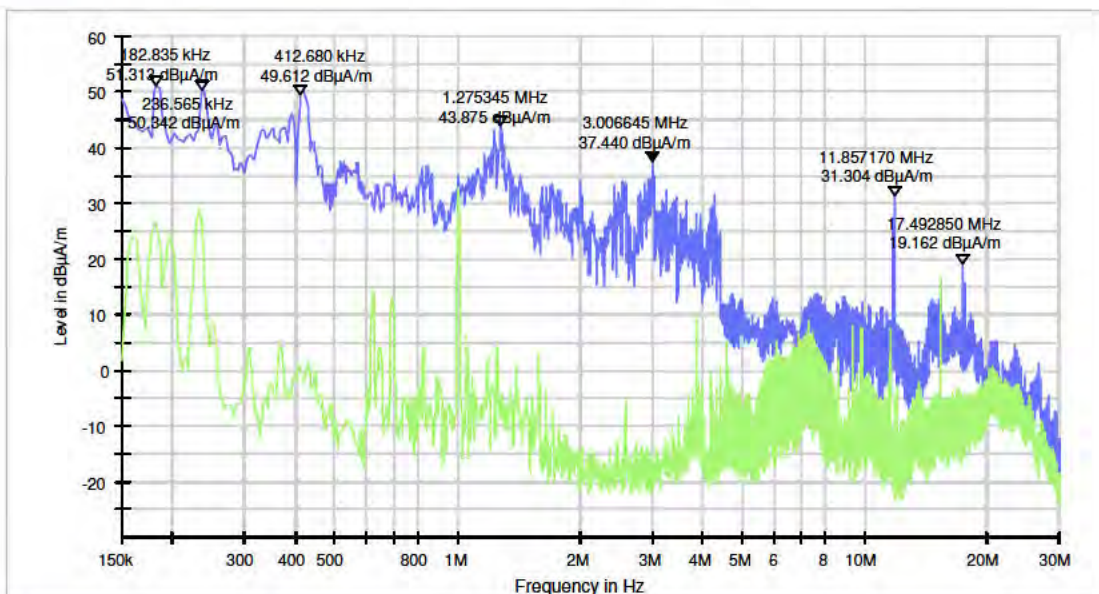
PK+_MAXH PK+_MAXH(1)@M2a ambient 150k - 30M
