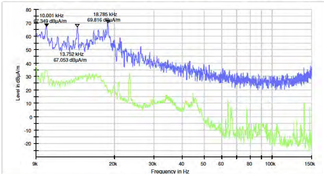
PK+_MAXH PK+_MAXH(1)@Ambient 9k-150k
