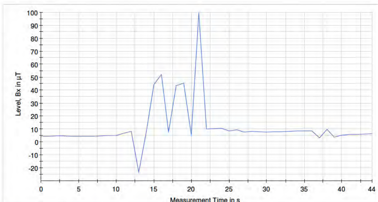
— Transit@70cm-Bx_M26
