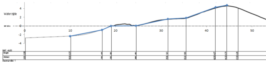
Figuur 31 voorbeeld schematisatie dijkwandprofiel t.b.v. oploopp- en overslagberekeningen (uit SH Hoogte, figuur 5.3)
