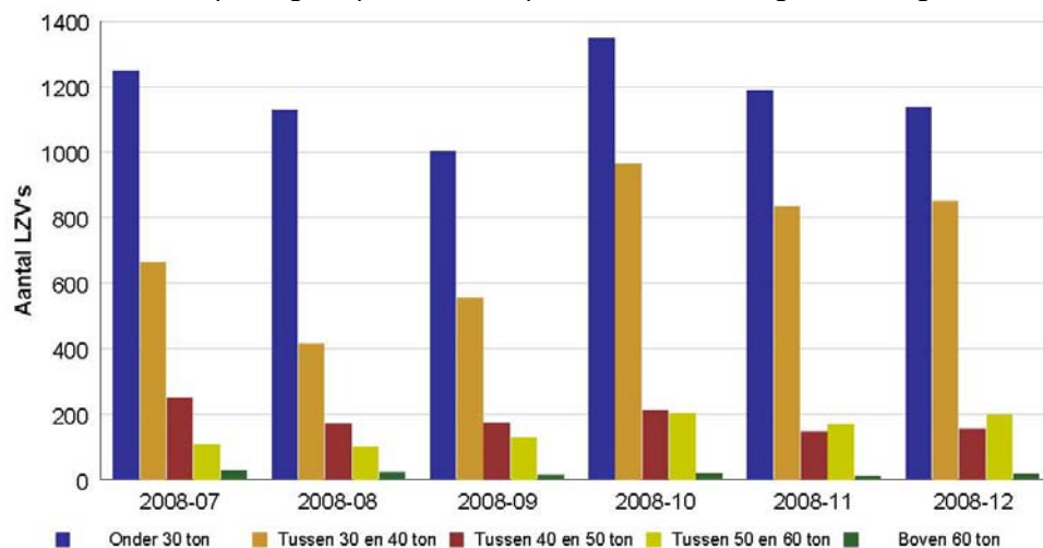
Grafiek 3.1 LZV-passages op WIM-VID-punten naar totaalgewicht, figuratief
