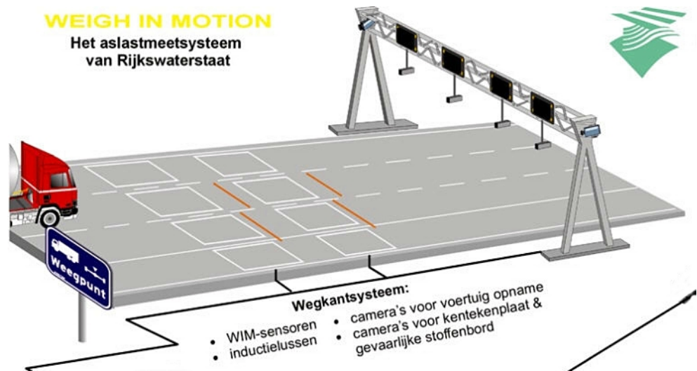
tekening 1: overzichtbeeld WIM –meetpunt
